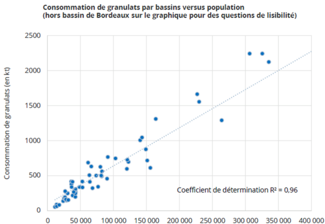
Figure 6 : Corrélation entre la consommation de granulats et la population Source : CERC Nouvelle-Aquitaine ; UNICEM ; INSEE
