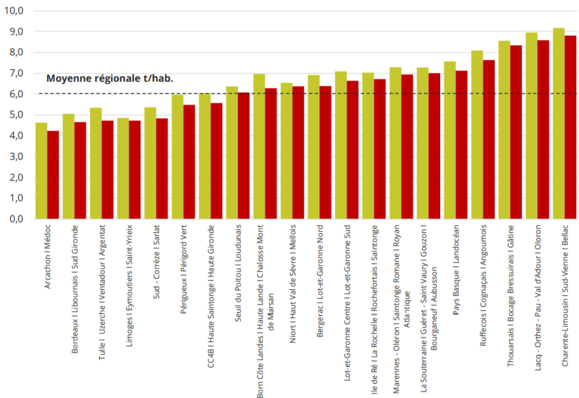
Figure 26 : Comparaison du ratio de consommation de granulats par pôle de consommation entre 2015 et 2035 en Nouvelle-Aquitaine en regard de l'évolution démographique, du développement de la construction bois et du recyclage Source : CERC Nouvelle-Aquitaine
