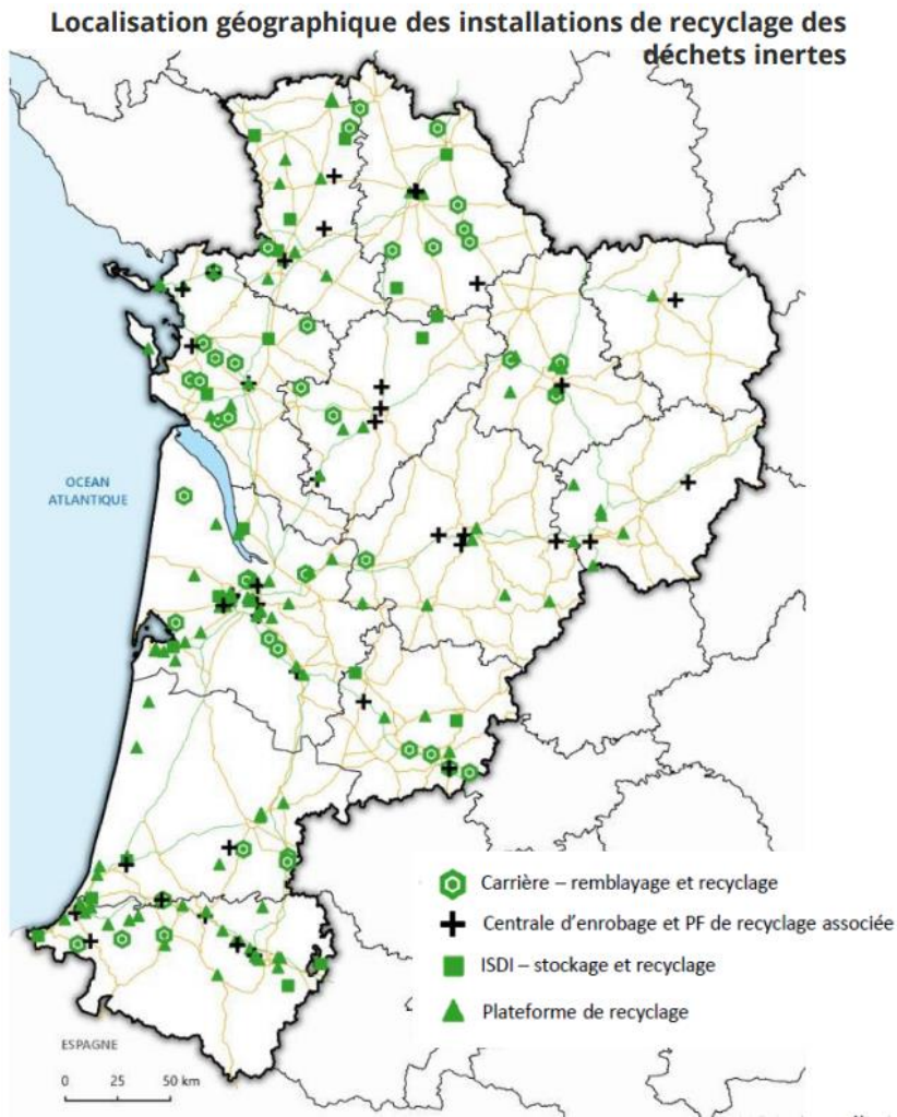
Figure 20 : Localisation des installations de recyclage de déchets inertes en Nouvelle-Aquitaine Source : CERC Nouvelle-Aquitaine
