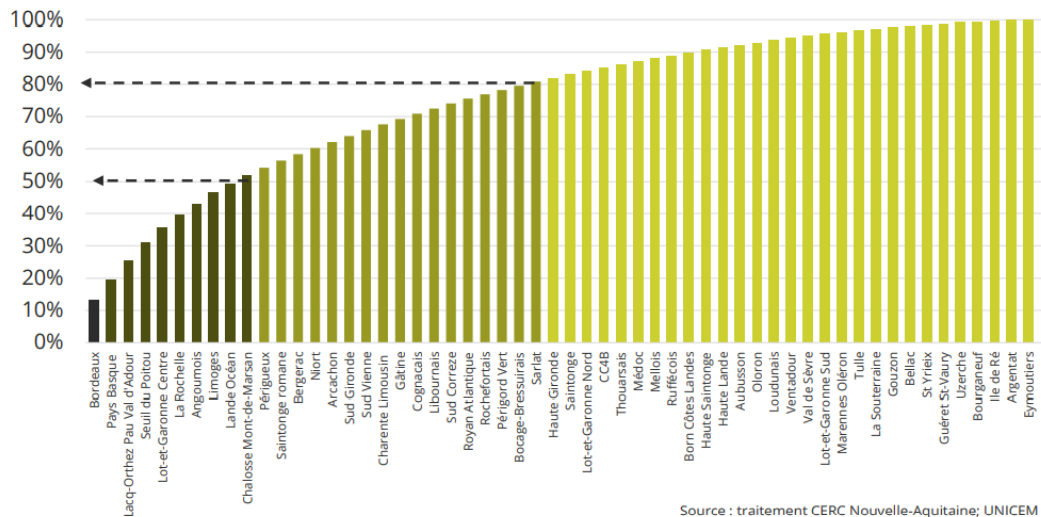
Figure 3 : Répartition de la consommation des 56 bassins par rapport à la consommation totale de granulats de la région Nouvelle-Aquitaine (en cumul) Source : CERC Nouvelle-Aquitaine ; UNICEM
