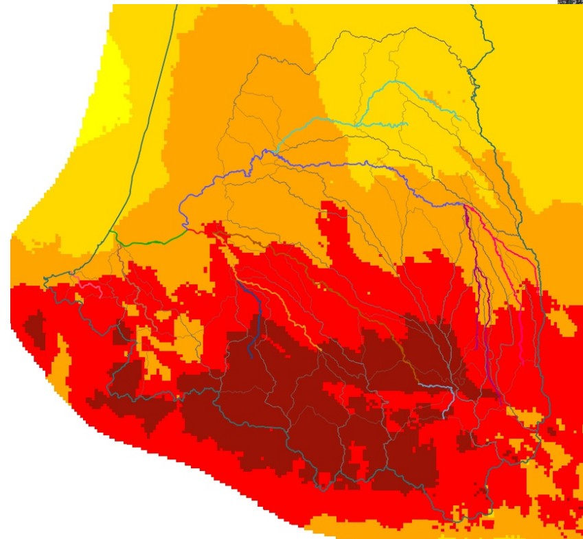
Cumul Pluie Antilope 72h du 26 janvier 2014 6h TU
