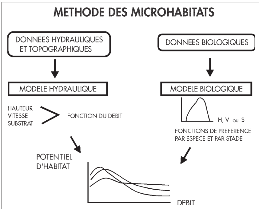
Fig. 2 - Principe de la méthode des microhabitats
