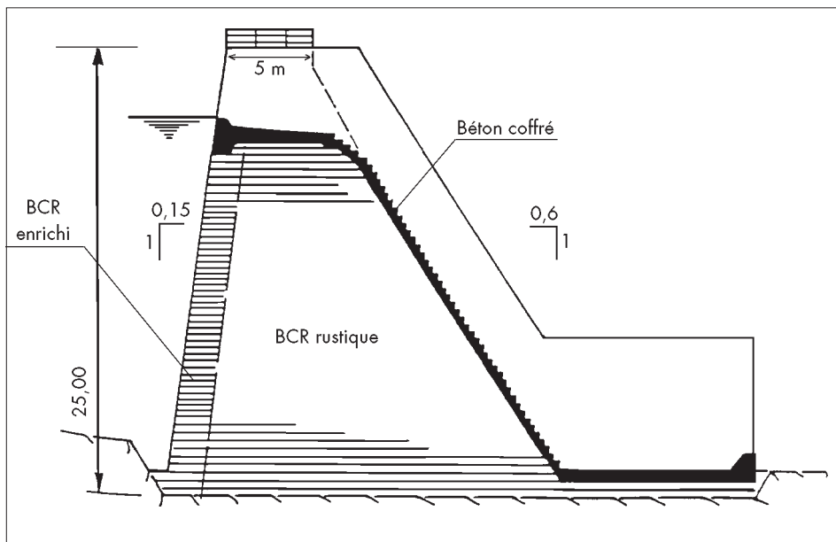
Fig. 6 - Barrage de LOUBERIA
