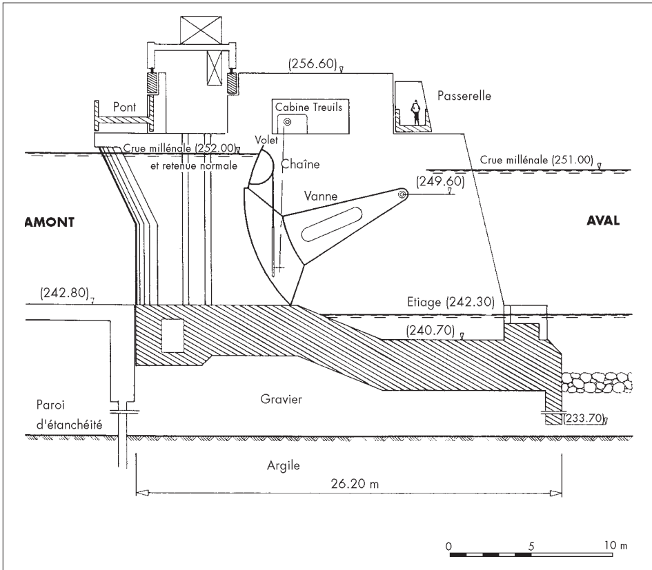
Fig. 9 - Barrage avec vanne segment
