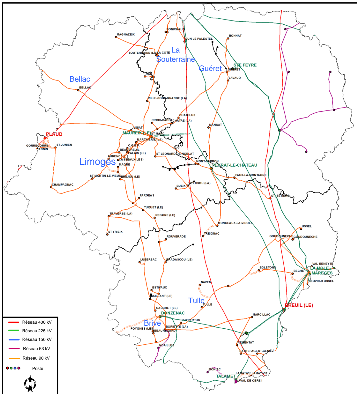
Le réseau de transport, les postes sources ERDF et les postes client actuels
