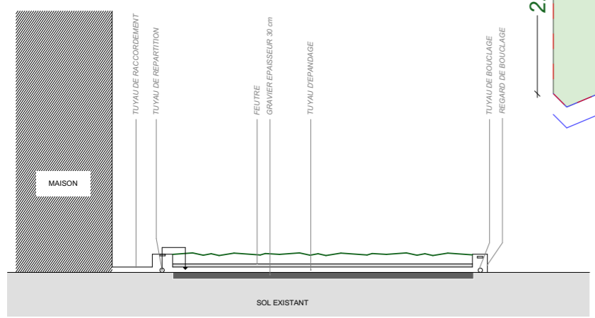
SCHEMA DE PRINCIPE Coupe Longitudinale
