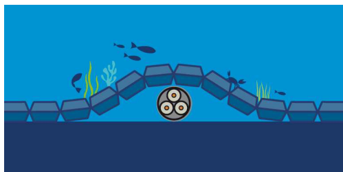
Matelas
