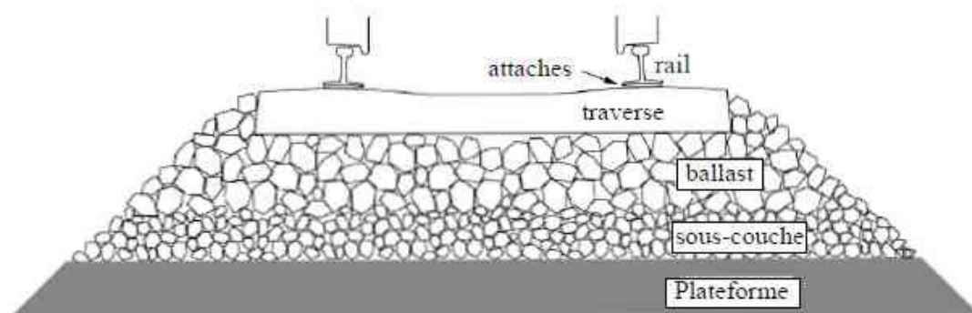
Illustration 24 - Coupe d'une voie ferrée (Quezada, 2014)
