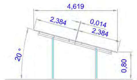
Figure 7 : Vue en coupe d'une table pour les Scénarios 1 et Scénario 2, variante 2.
