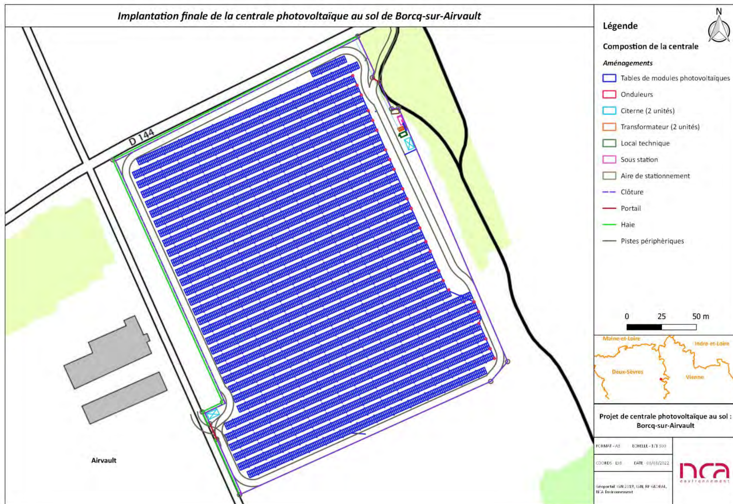
Figure 63 : Plan de masse du projet à l'échelle du périmètre sous emprises
