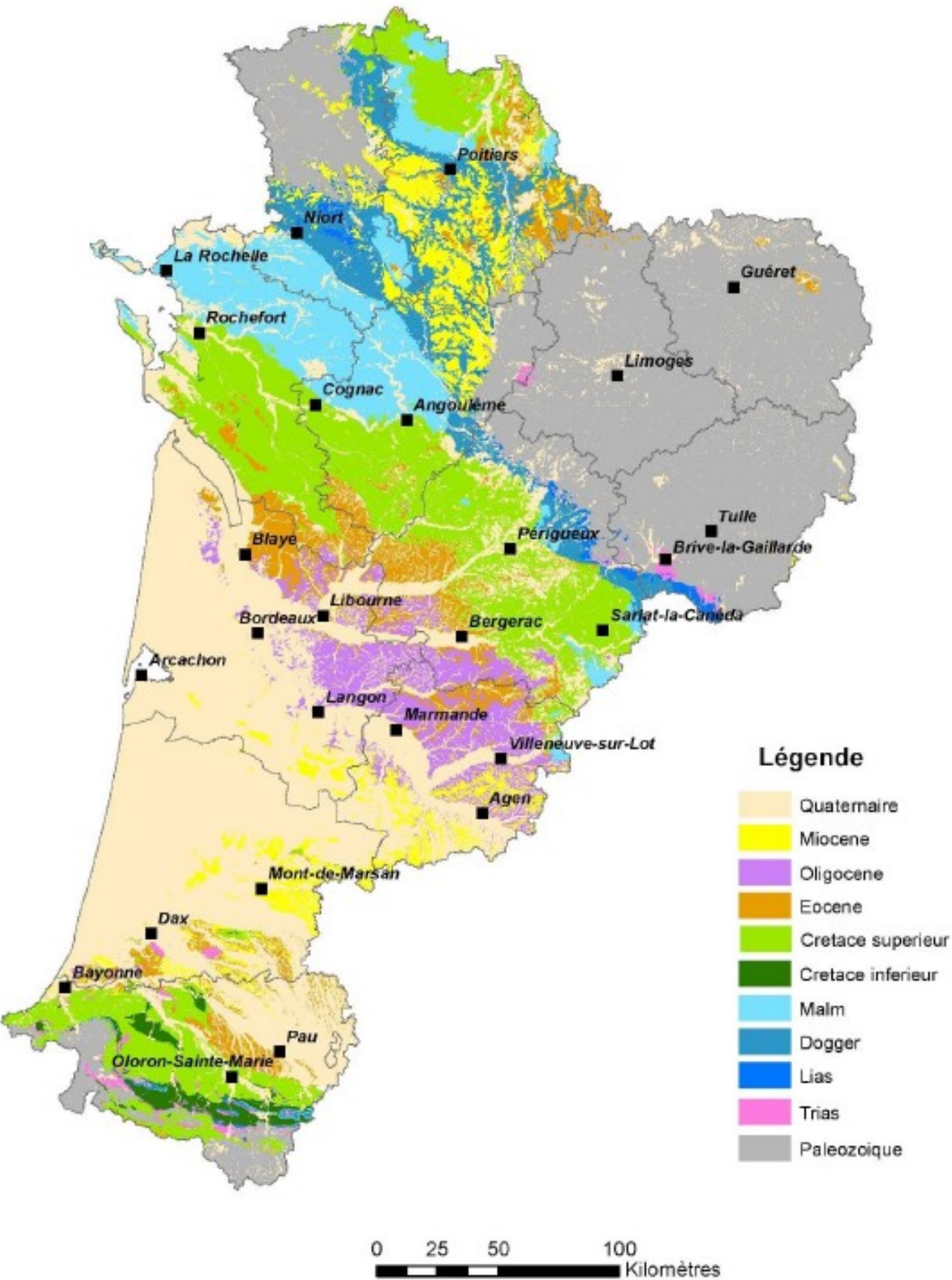
Illustration 16 -Carte géologique simplifiée de la Nouvelle-Aquitaine
