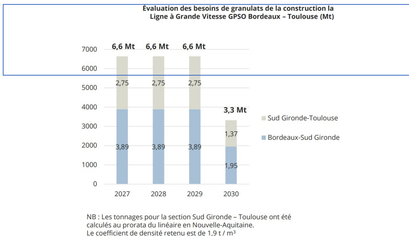
Figure 30 : Répartition du besoin en granulats exceptionnel au regard du projet ferroviaire de ligne à grande vitesse Bordeaux-Toulouse Source : CERC Nouvelle-Aquitaine ; SNCF réseau ; EGIS
