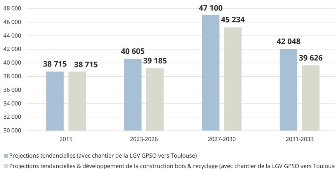
Figure 33 : Synthèse des besoins en granulats en regard de l'évolution démographiques, du développement de la construction bois, du développement du recyclage et du projet de ligne ferroviaire à grande vitesse Bordeaux-Toulouse Source : CERC Nouvelle-Aquitaine
