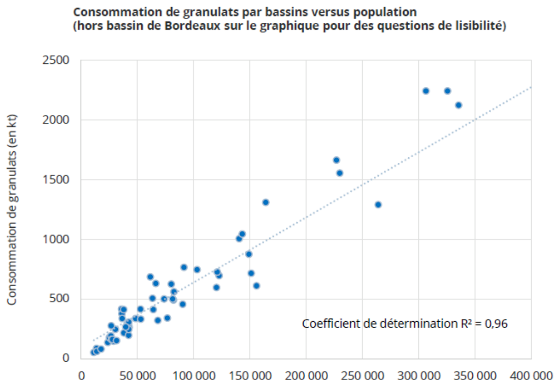
Figure 6 : Corrélation entre la consommation de granulats et la population Source : CERC Nouvelle-Aquitaine ; UNICEM ; INSEE
