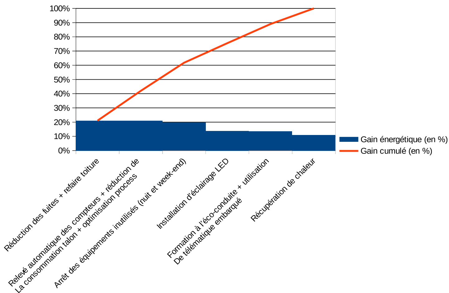
Illustration 7 : Contributions des 20 principales préconisations vertueuses* au potentiel cumulé d'économie de 7 384 MWh/an
