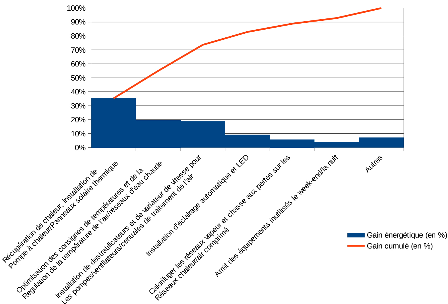
Illustration 7 : Contributions des 52 principales préconisations vertueuses* au potentiel cumulé d'économie de 21 876 MWh/an
