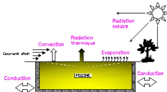
Figure 2.1 : Représentation des pertes thermiques au travers d'une piscine (source : thermexcel.com)
