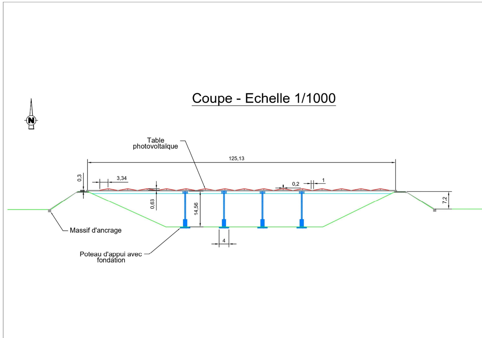
Figure 2 Schéma de la structure – vue de coupe (source : Ventelys)
