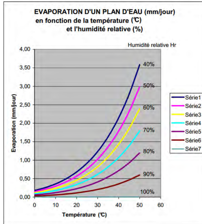
Figure 2.2 : Taux d'évaporation d'un plan d'eau en fonction de la température et de l'humidité relative (source : enseeiht.fr)
