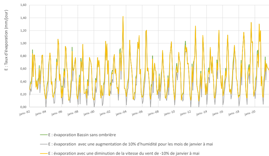
Figure 4.3 : Effet de la diminution de la vitesse du vent et de l'augmentation de l'humidité
