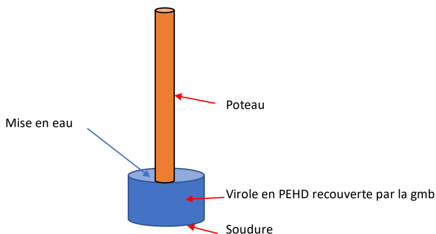
Schéma du dispositif de contrôle de l'étanchéité autour des poteaux
