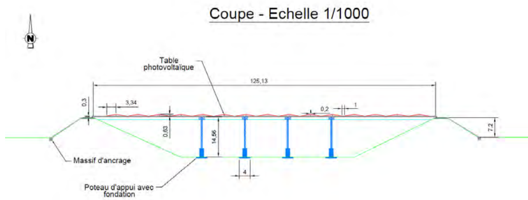
Figure 3.2 : Coupe de principe de la structure projetée (Doc. Ventelys)
