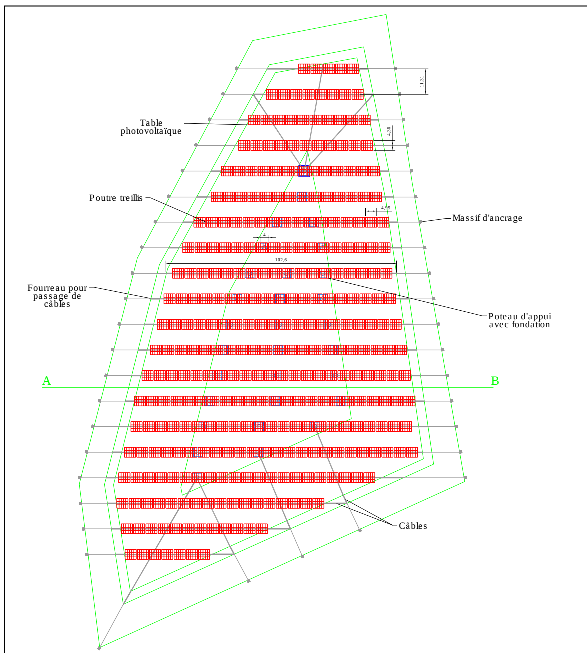
Figure 1 : Schéma de principe de la structure (source : Ventelys)
