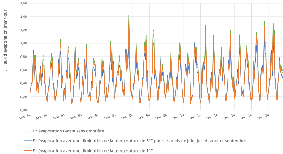
Figure 4.2 : Effet de la diminution de température sur l'évaporation
