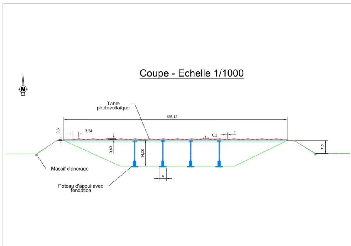
Figure 2 : Schéma de principe de la structure – vue de coupe (source : Ventelys)
