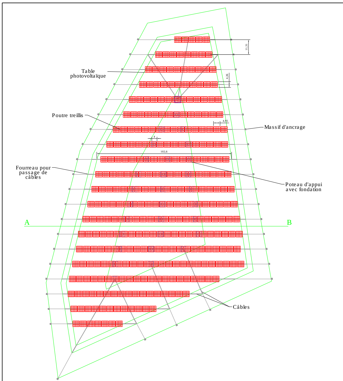
Figure 2 : Schéma de principe de la structure (source : Ventelys)
