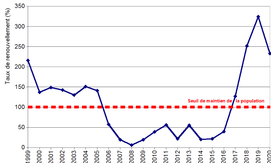
Evolution du taux de renouvellement de la population de grande alose estimée dans le bassin Garonne-Dordogne
