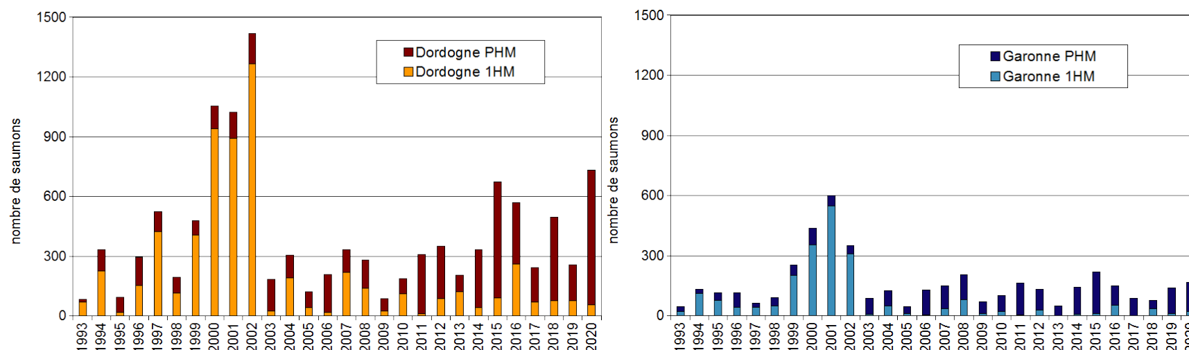
Evolution des comptages de saumons atlantiques de 1 (1H) et plusieurs (PHM) hivers de mer au niveau de Tuilières (Mauzac pour les années 2006-2008) sur la Dordogne et Golfech sur la Garonne (source : MIGADO)
